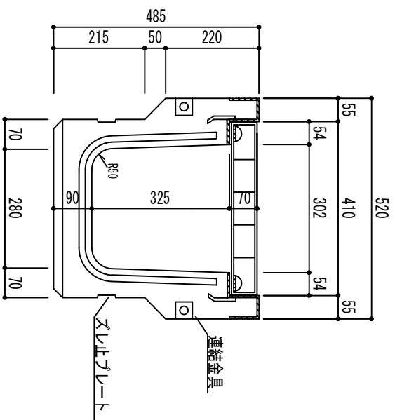
断面図
