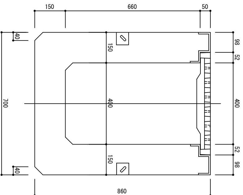
断面図
