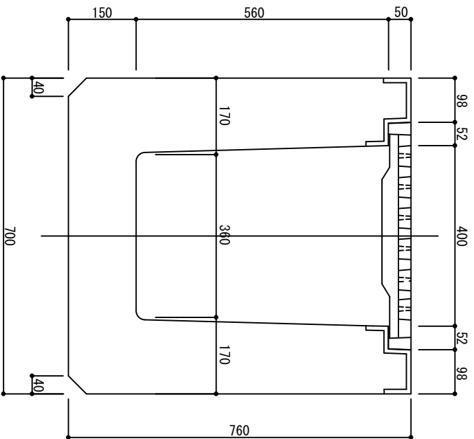
断面図
