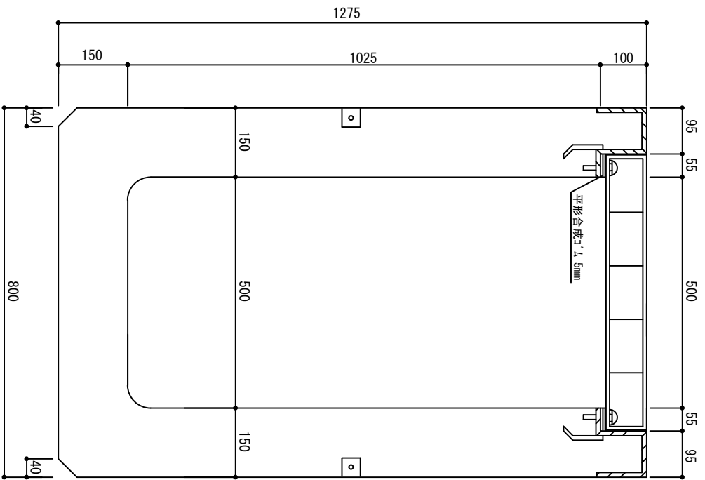
断面図
