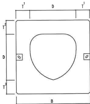
寸法表
