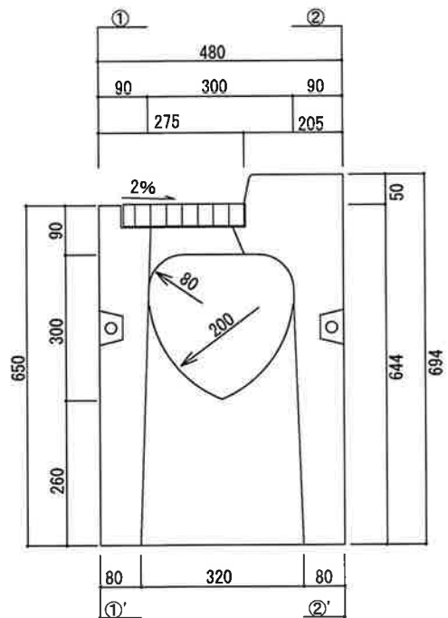
断面図
