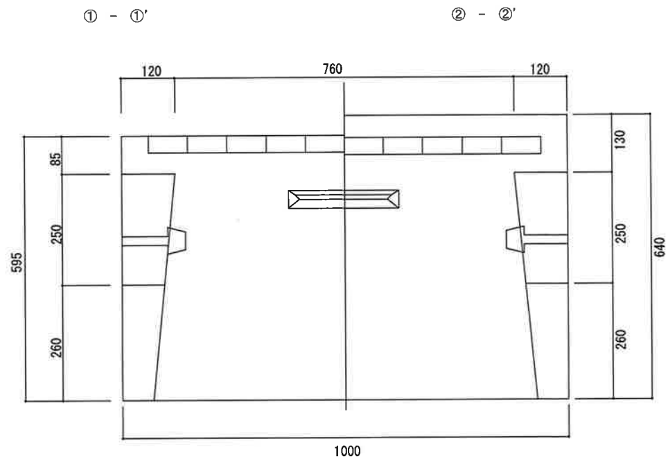
側面図
