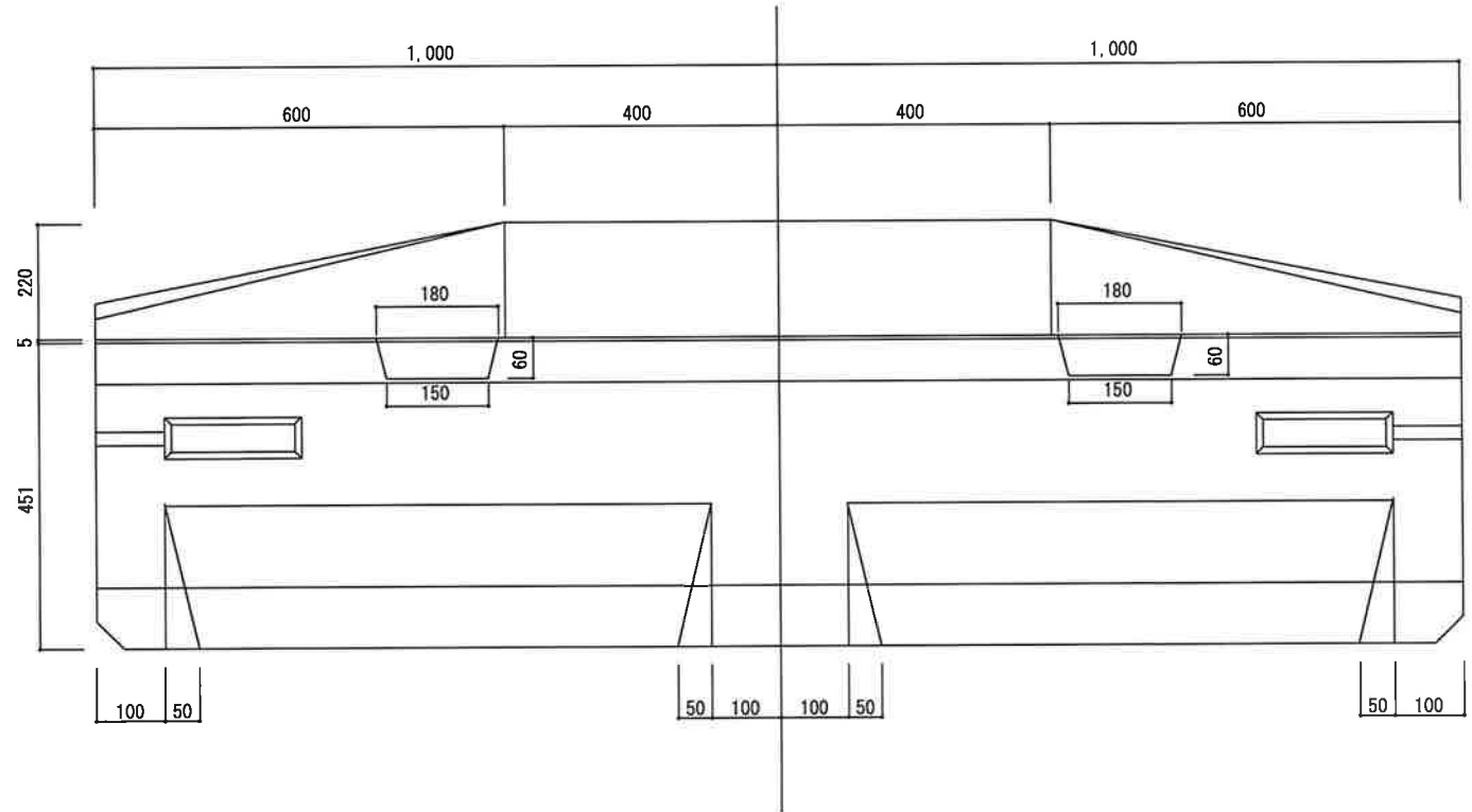
側面図
