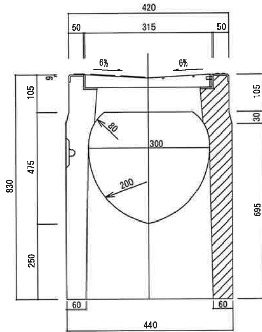
断面図
