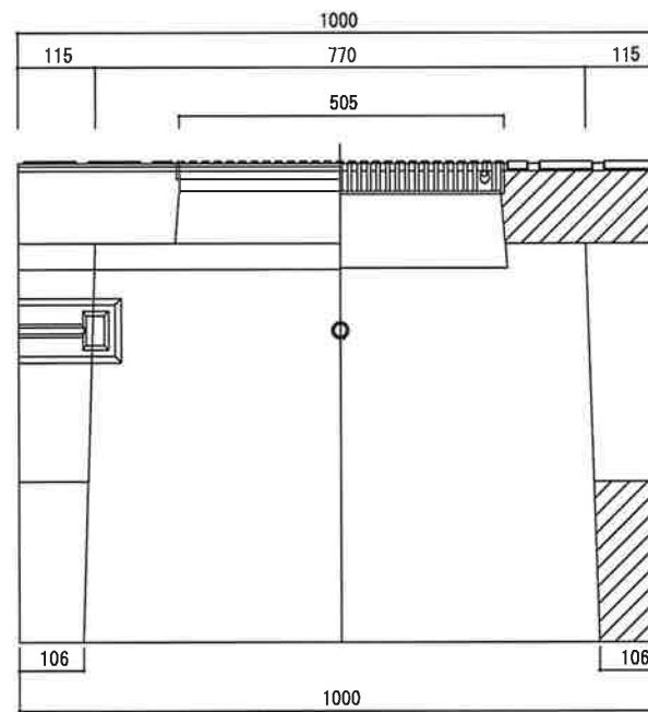
側面図
