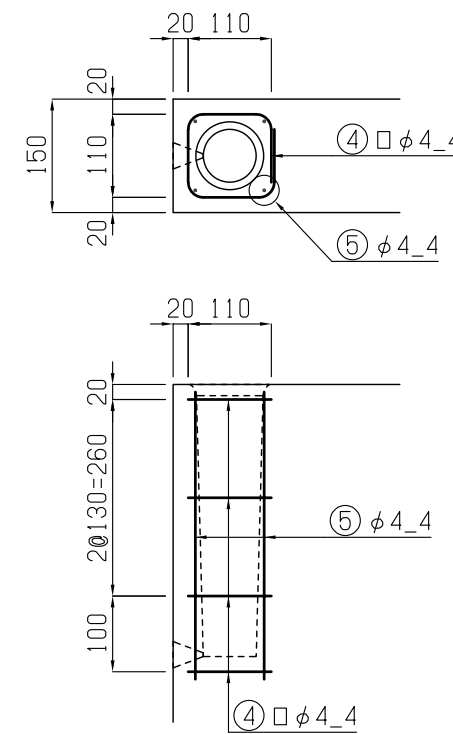
支柱用孔部配筋図 S=1:10
